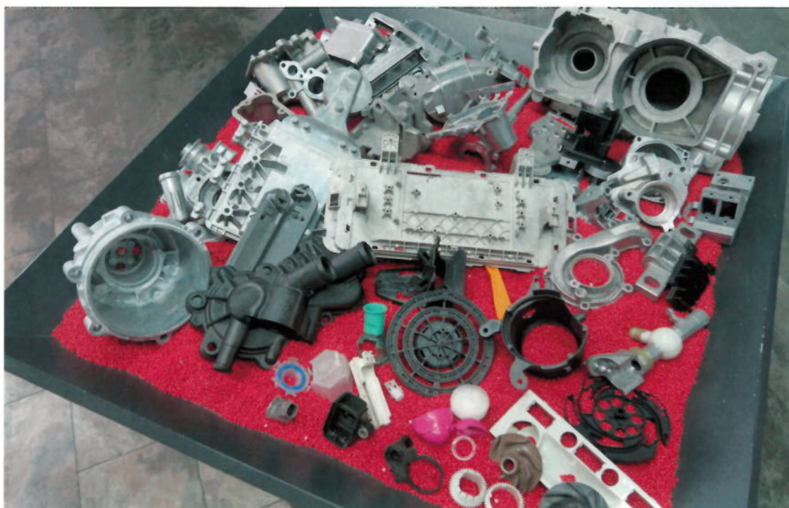
Bild 5: Das Produktions- programm von appex umfasst Formen sowohl für Druckguss- prototypen als auch für Spritz- gussprototypen
