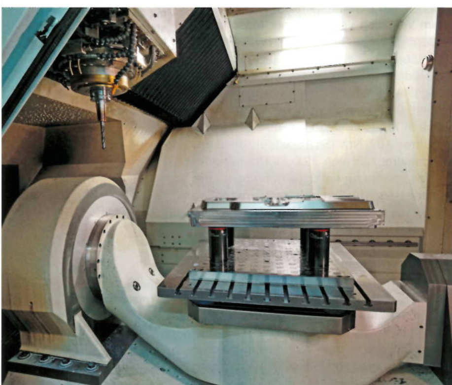
Bild 8: Blick in den Arbeitsraum mit einem auf einer Wechselpalette montierten Werk- stück
