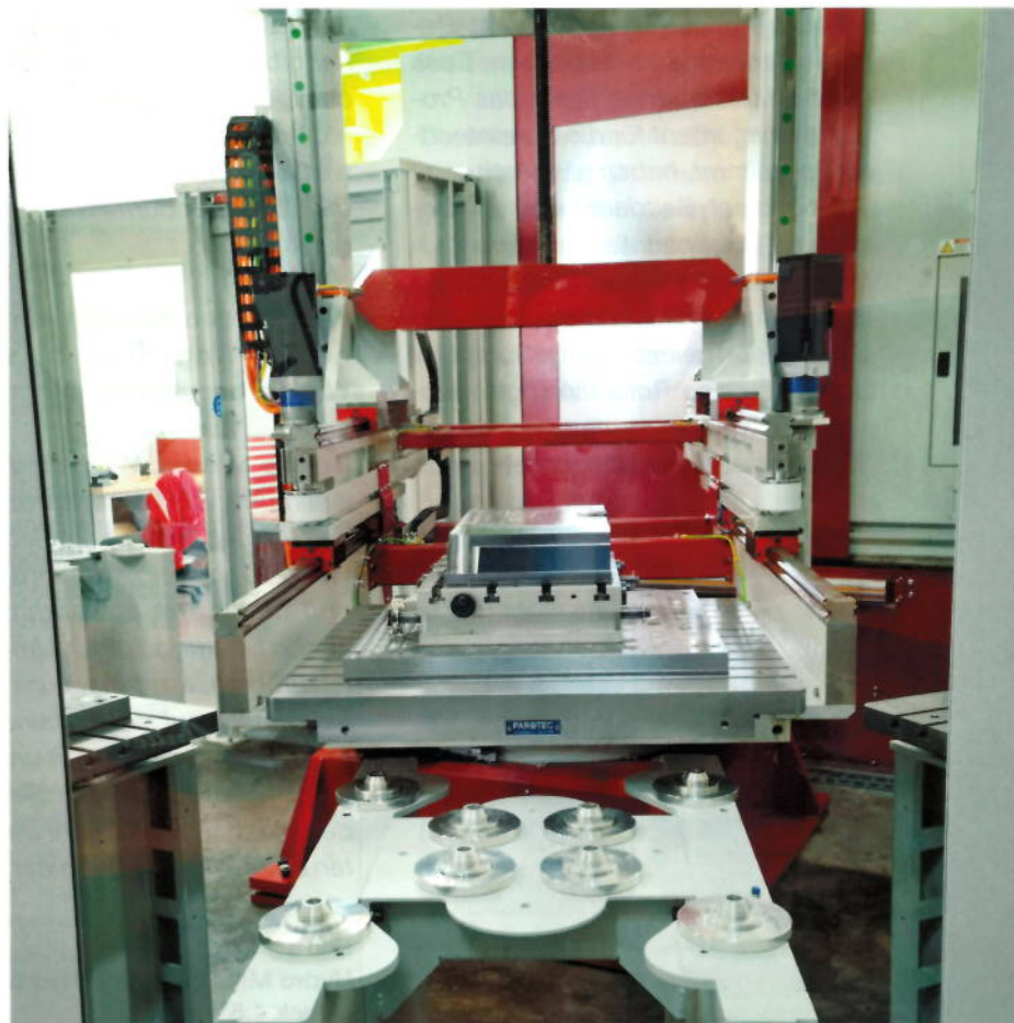
Bild 10: Die Automation RCH2 bewältigt Nutzlasten bis zu 1.500 kg (Bilder 6 bis 8, 10: Klaus Vollrath)
