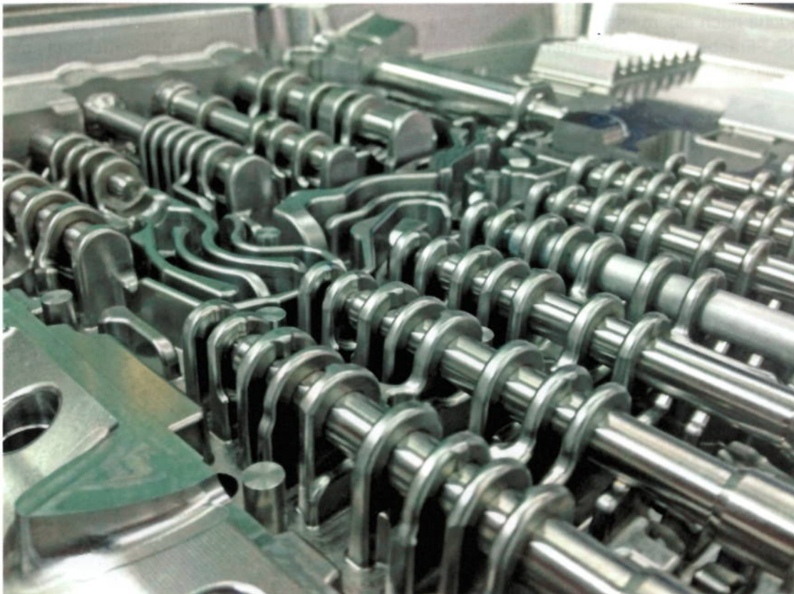
Bild 3: Bei appex aus Stahl gefräste Druckgießform für das Labyrinthgehäuse eines Automatikgetriebes
